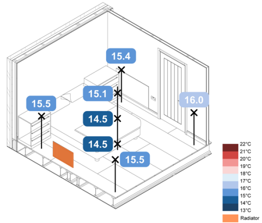
-5°C Loft ASHP Rads + UFH SAP – Air - 7h
